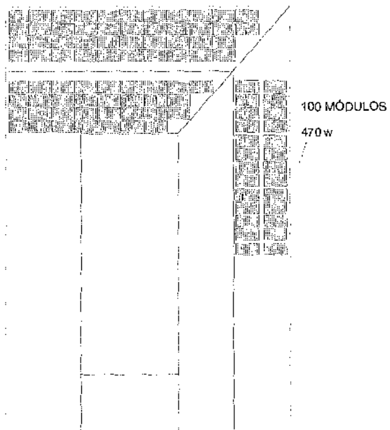
4 VISTA SUPERIOR DOS MÓDULOS
